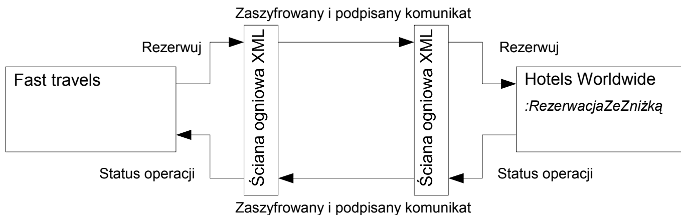
Rysunek 2. Zabezpieczona wymiana komunikatów SOAP.
